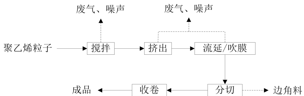
图 2.6.1 生产工艺及产污环节图
