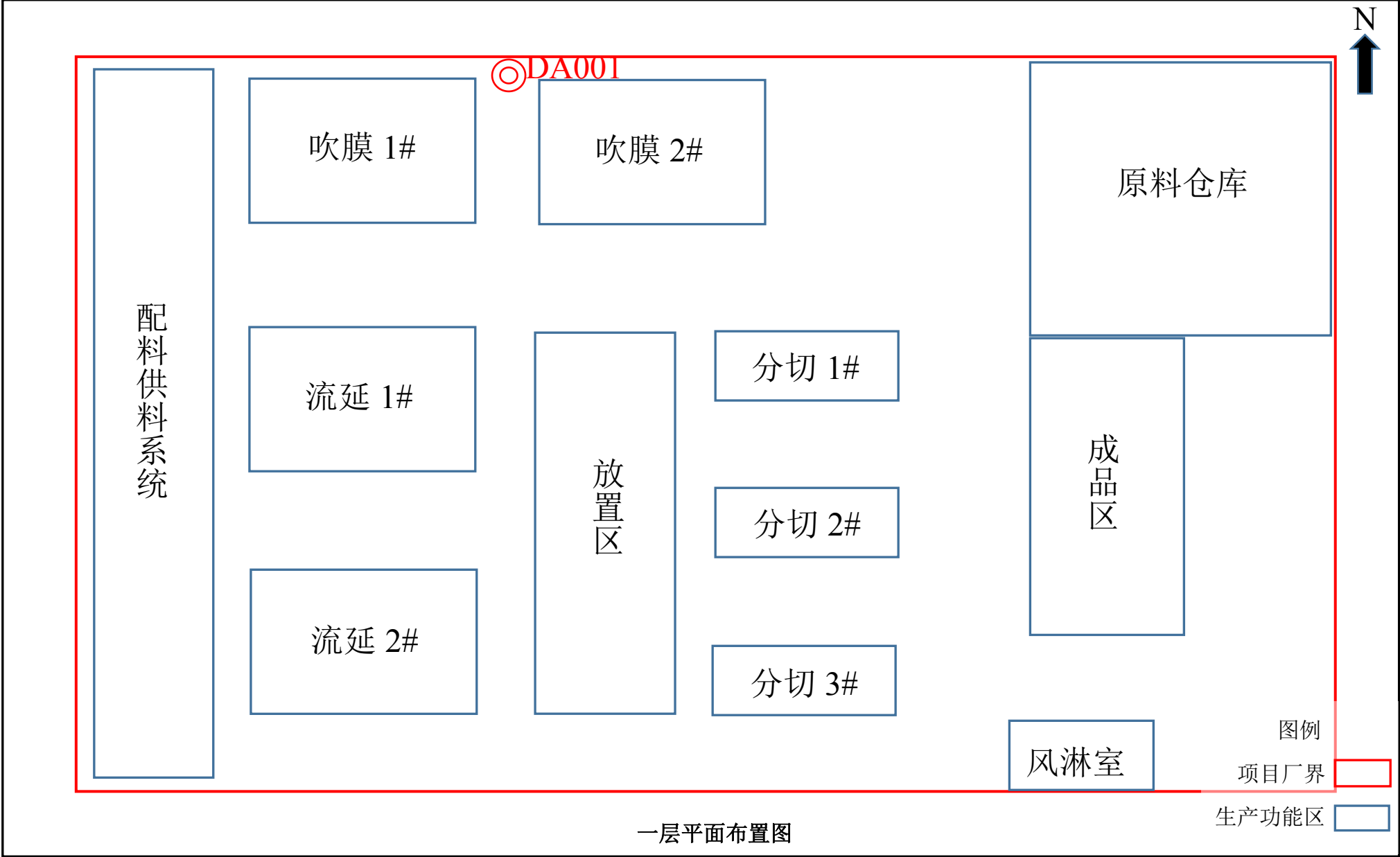
附图 4 平面布置图
