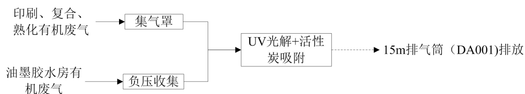
图 4.2.1 本项目废气处理工艺
