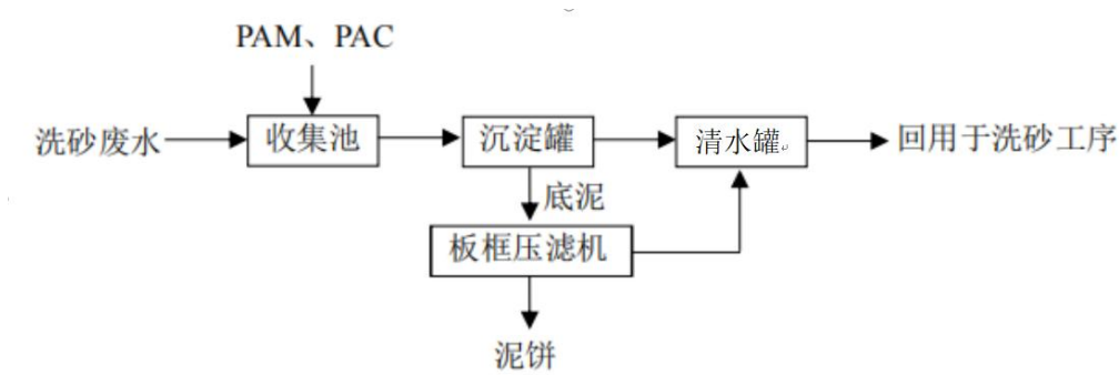
图 4.3-1 洗砂废水处理工艺流程图
